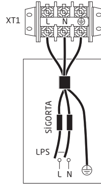
MONOFAZE DIŞ ÜNİTE GÜÇ KAYNAĞI
